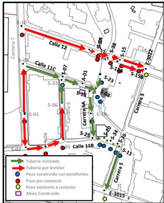
Figura 7. Localización de las obras de alcantarillado sanitario objeto de este contrato en el barrio Rumipamba
