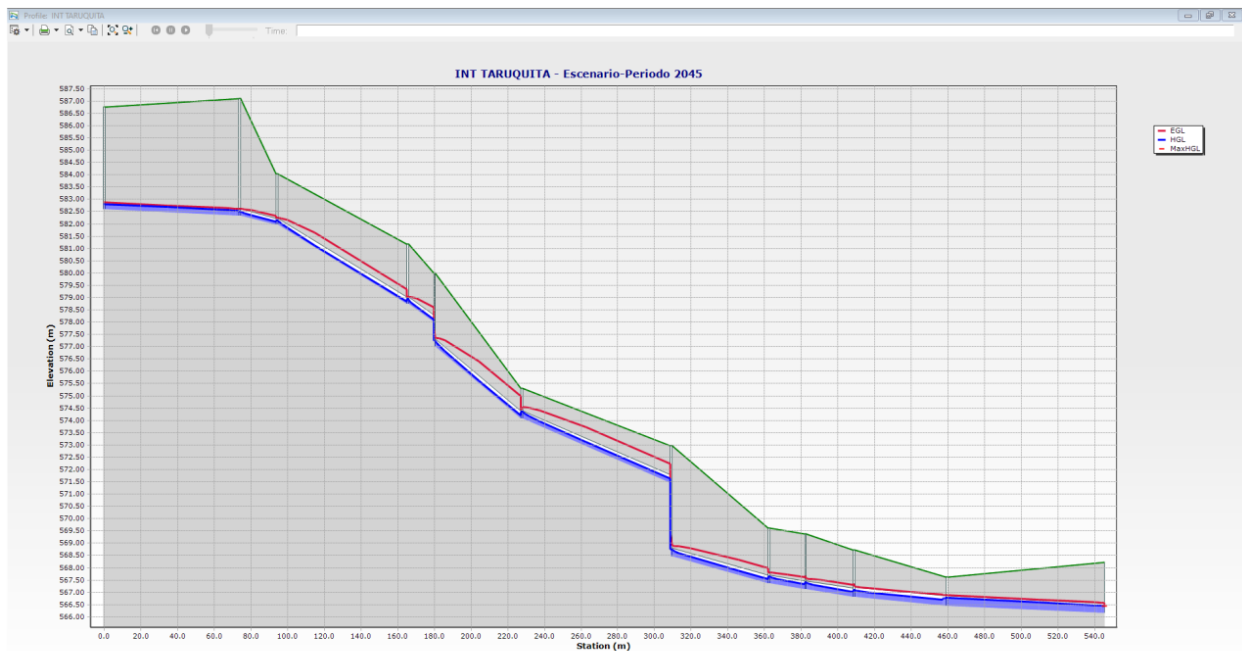
Figura 13. Perfil hidráulico del colector Taruquita
