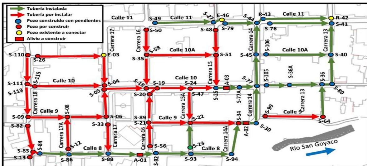
Figura 3. Localización de las obras de alcantarillado sanitario objeto de este contrato en el barrio Huasipanga
