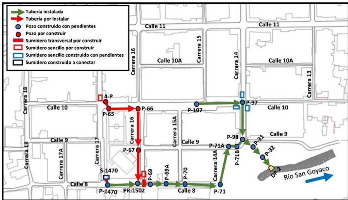
Figura 4. Localización de las obras de alcantarillado pluvial objeto de este contrato en el barrio Huasipanga
