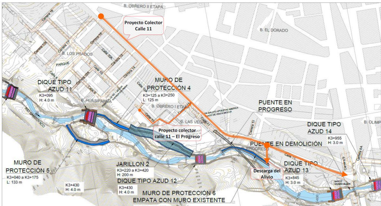
Figura 10. Localización de las obras de alcantarillado completo calle 11.
